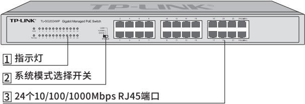
图1-6 TL-SG2024MP前面板示意图
